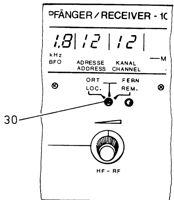
Bild 2.43 Ort/Fern-Schalter
