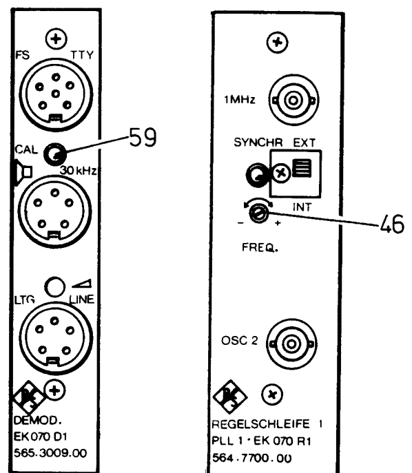
Bild 2.19 Frequenzkalibrierung
