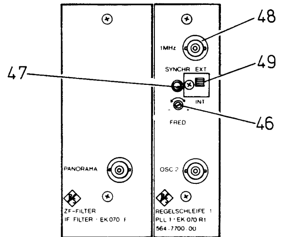
Bild 2.29 Normalfrequenzanschluß
