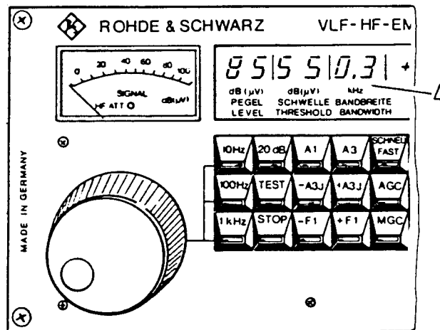
Bild 2.10 Bandbreitenanzeige
