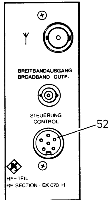
Bild 2.23 Steueranschluß
