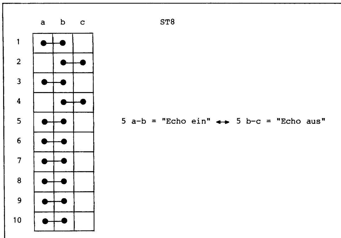
Bild 2.45 Kurzschlußstecker in Stellung "Echo ein"
